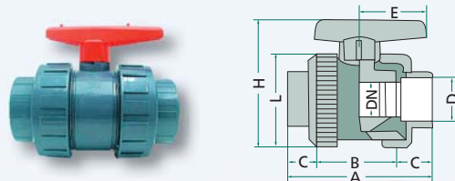
Rozměry (mm)
