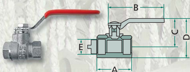
Rozměry (mm/coul)
